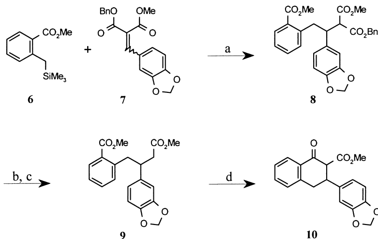
Scheme 2. (a) CsF, HMPA, 60 °C; (b) \text{H}_2 , 10% Pd/C; (c) 150 °C; (d) NaOMe/MeOH/THF.
